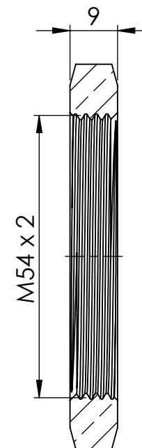
SCHNITT A-A
